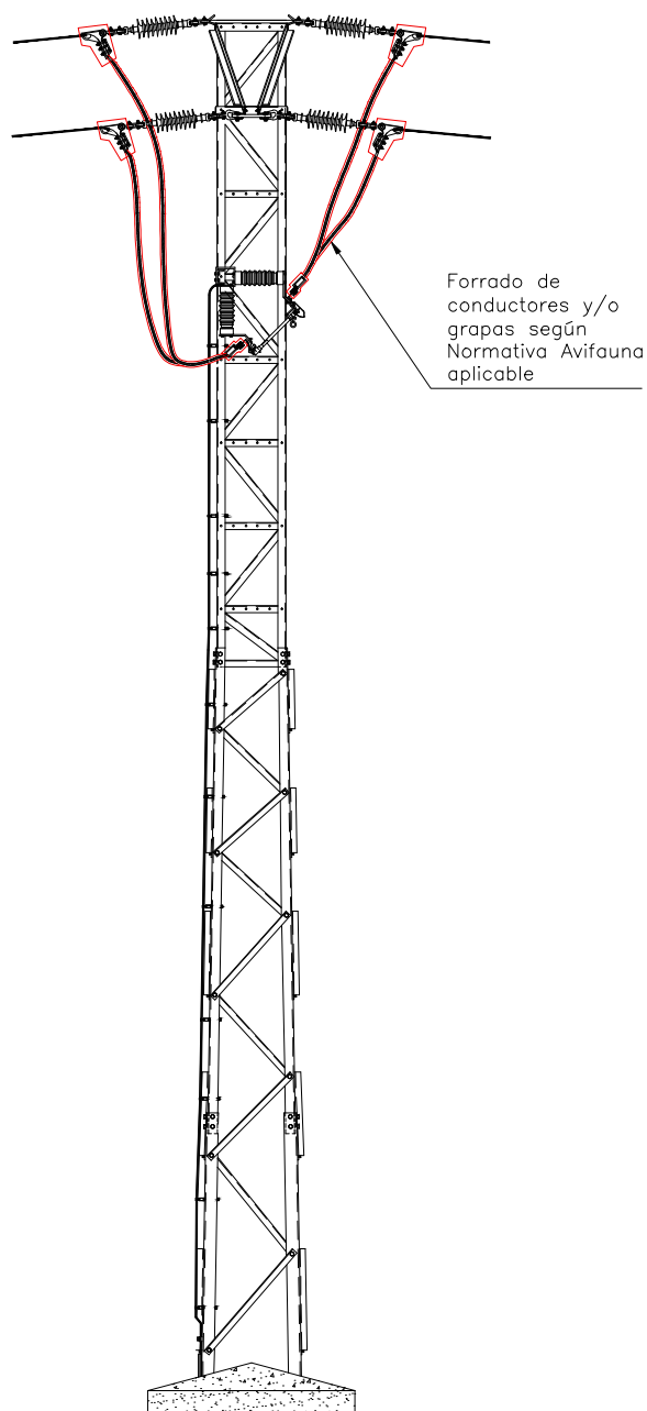
VISTA LATERAL
